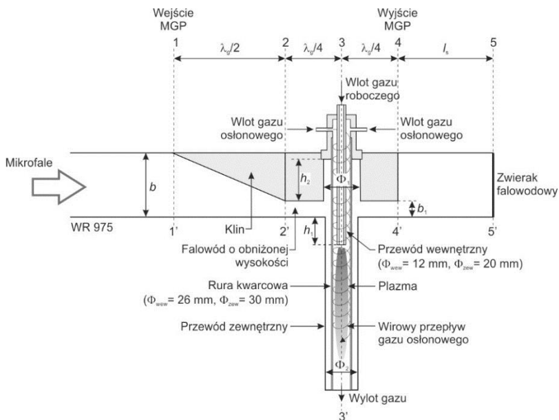
Rys. 1. MGP o strukturze współosiowej [Mizeraczyk i in. 2012]
