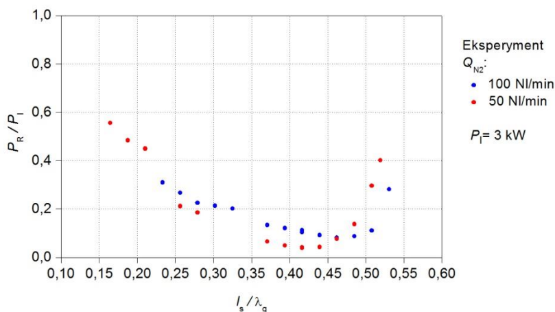
Rys. 2. Zmierzone charakterystyki elektrodynamiczne MGP
